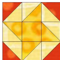
Dubbele vriendskapster
