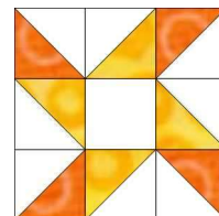
Eksentrieke Ster
