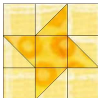
Vriendskapster
